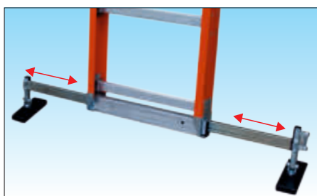
Basetta stabilizzatrice a scomparsa si richiude con sfilo telescopico su entrambi i lati per facilitare il trasporto ed è dotata di piedini basculanti che si adattano autonomamente all'inclinazione del suolo
