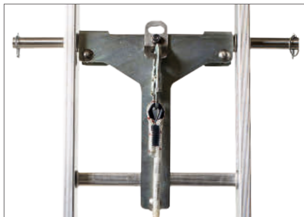
Piastra di fissaggio superiore con punto ancoraggio dotato di moschettone e tubo Ø 25 mm. per rinforzo gradino
