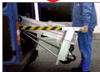
E' possibile ripiegare le barre di sostegno mediante dispositivo con sblocco rapido senza l'ausilio di utensili per consentirne il trasporto anche su piccoli automezzi.
