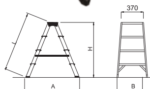
Gradino piano profondo mm. 80 con zigrinatura anti-scivolo
