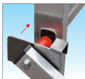
Traverse ad aggancio rapido con dispositivo anti-distacco
